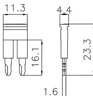
Zwieracz sprężynowy ZSN-4-2
