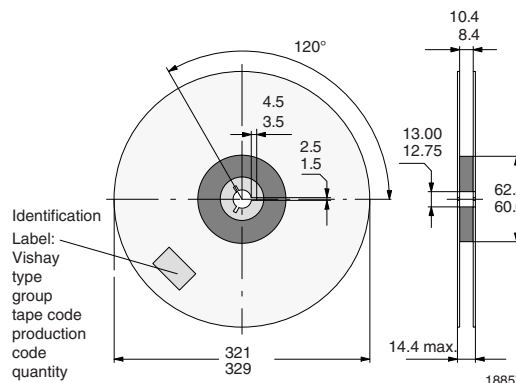
Fig. 12 - Reel Dimensions - GS18
