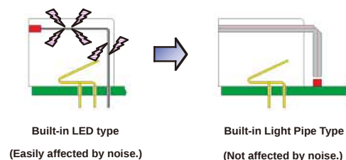
Fig.3 : EMI Protection
