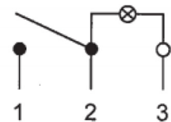
3P SPST OFF-ON (LED-D)
