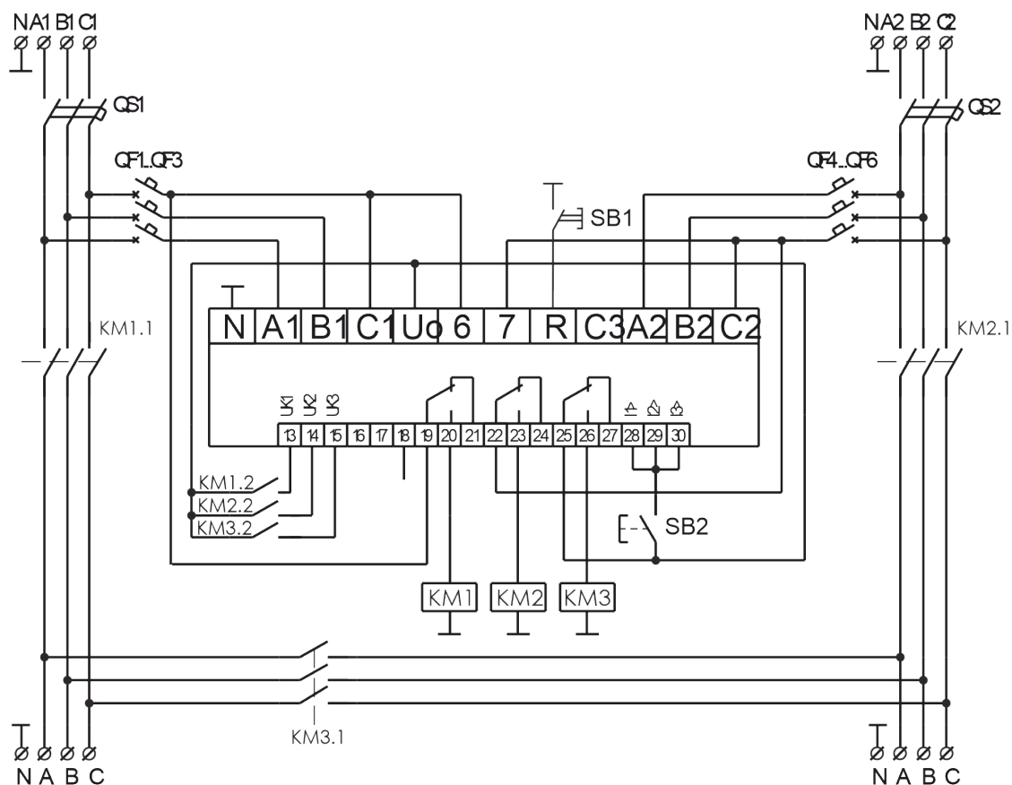
Rys. 11) Aplikacja N1 + N2 + S ze stycznikami
