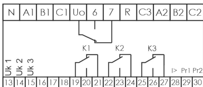
Rys. 1 Listwy łączeniowe sterownika
