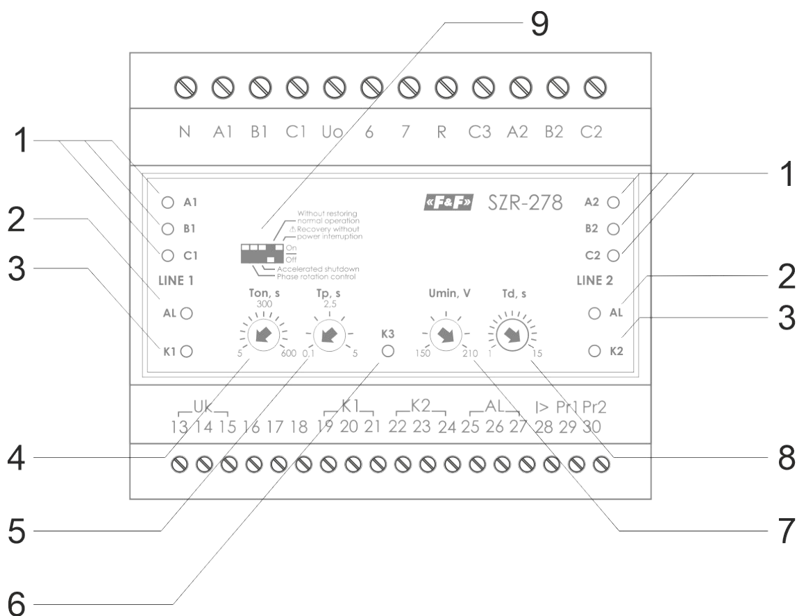
Rys. 7) Panel operatorski sterownika SZR-278
