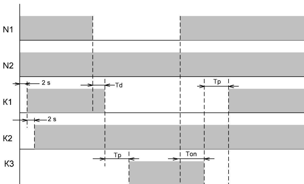
Rys. 6) Tryb N1 + N2 + S - diagram przełączeń
