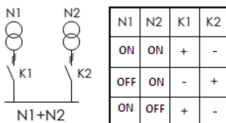
Rys. 3) Tryb N1 + N2 - schemat przełączeń
