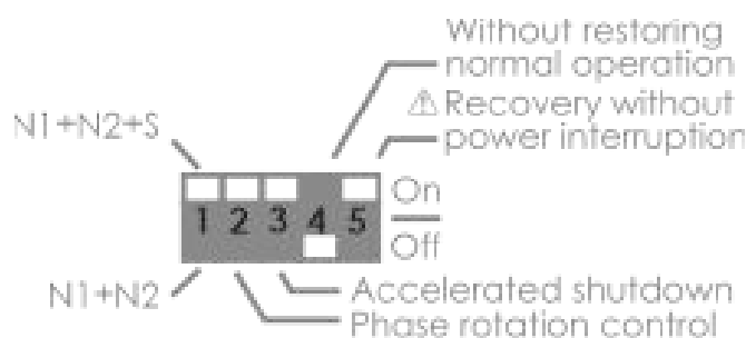
Rys. 8) Przełączniki konfiguracyjne
