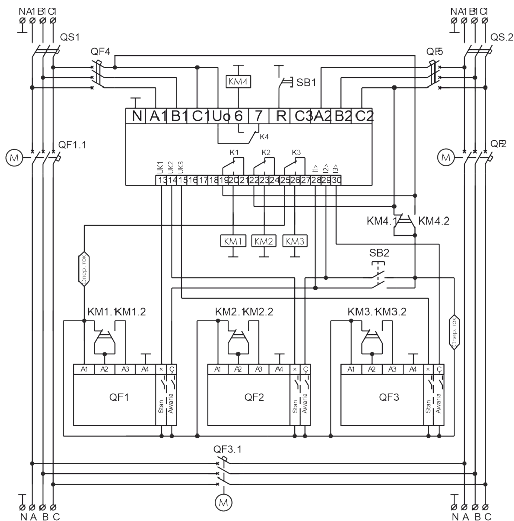
Rys. 12) Aplikacja N1 + N2 + S z wyłącznikami z napędem silnikowymi
