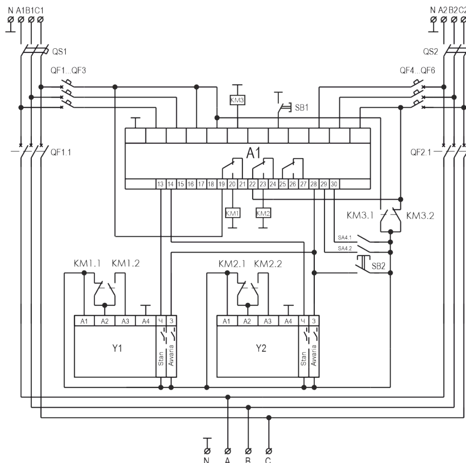
Rys. 10) Aplikacja N1 + N2 z wyłącznikami z napędem silnikowymi
