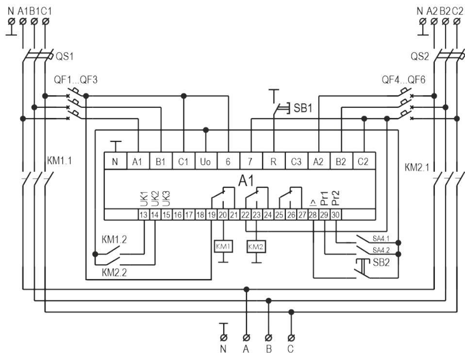
Rys. 9) Aplikacja N1 + N2 ze stycznikami
