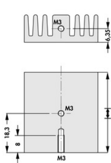
SK 126 25 2 x M 3 SK 126 37,5 2 x M 3
