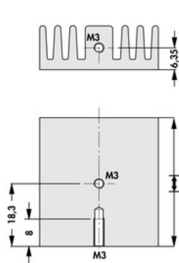
SK 126 25 2 x M 3 SK 126 37,5 2 x M 3
