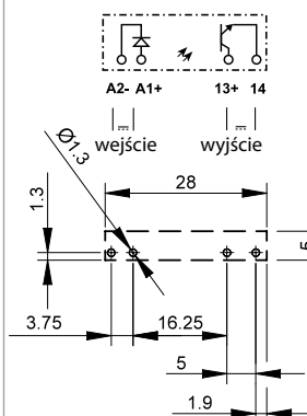
Rysunek otworów montażowych
