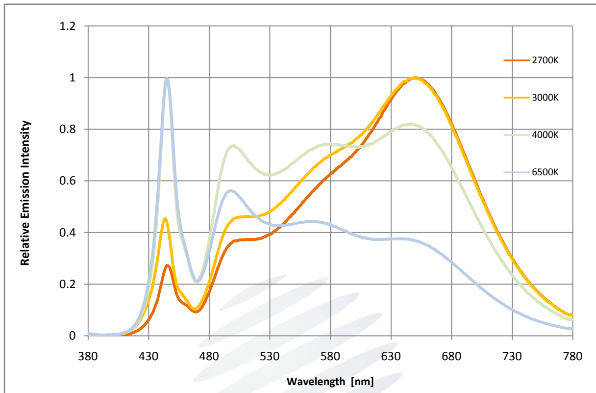
Fig 1-13 Spectrum Distribution 光譜分布特性曲线
