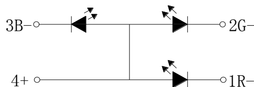
Fig.1-4 Polarity 极性
