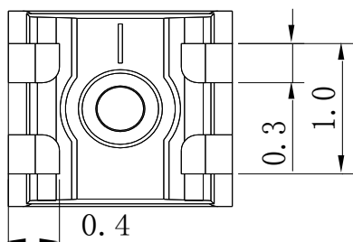
Fig.1-3 Bottom view 背面视图
