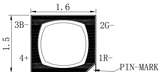
Fig.1-1 Top view 正面视图
