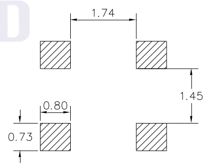
Fig.1-5 Pad 焊盘
