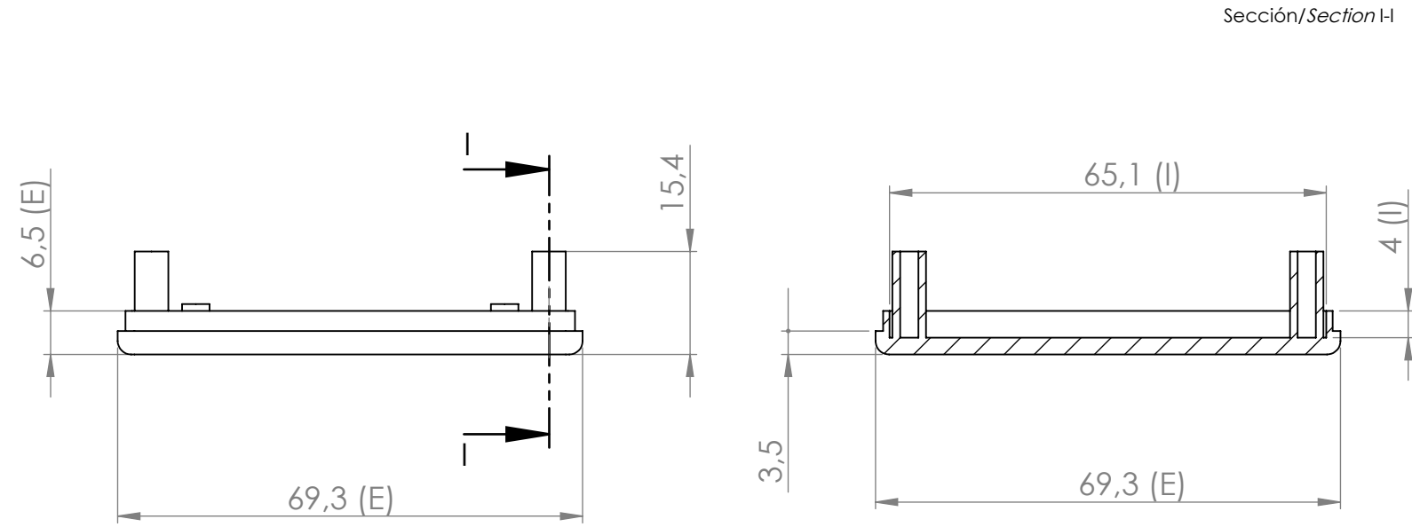
Sección/Section H
