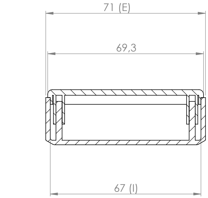
Sección/Section B-B
