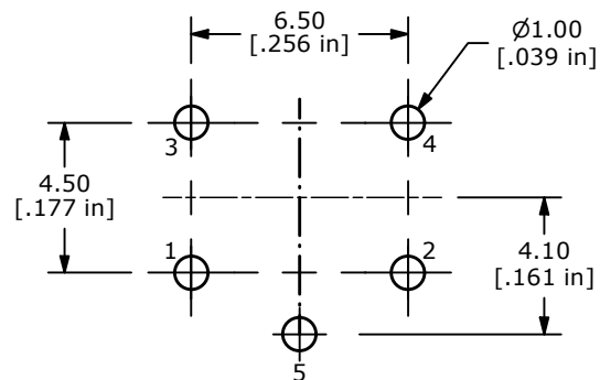
P.C. LAYOUT
