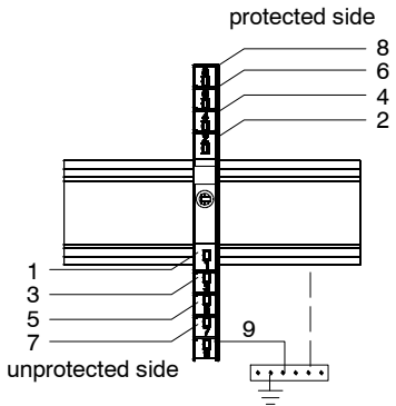
4 pole-version
