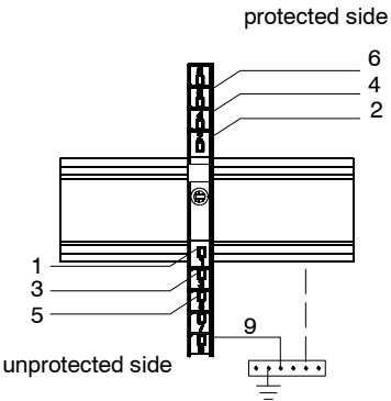
3 pole-version
