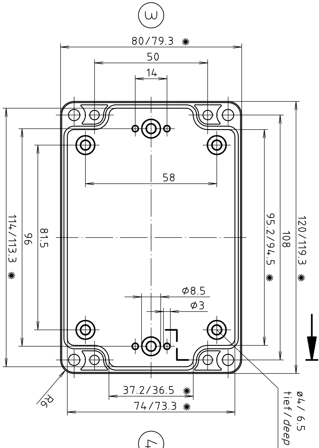
Unterteil/base
