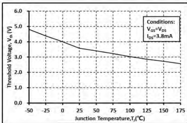
图. 9 阈值电压随温度变化曲线
