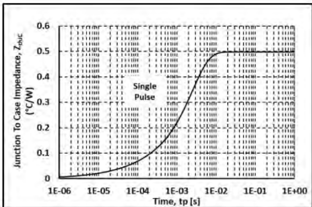
图. 23 热阻曲线
