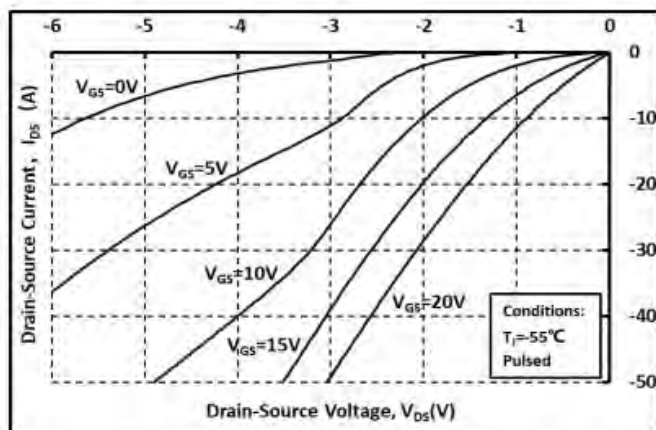
图. 13 第三象限曲线 @ T_j = -55^\circ\text{C}
