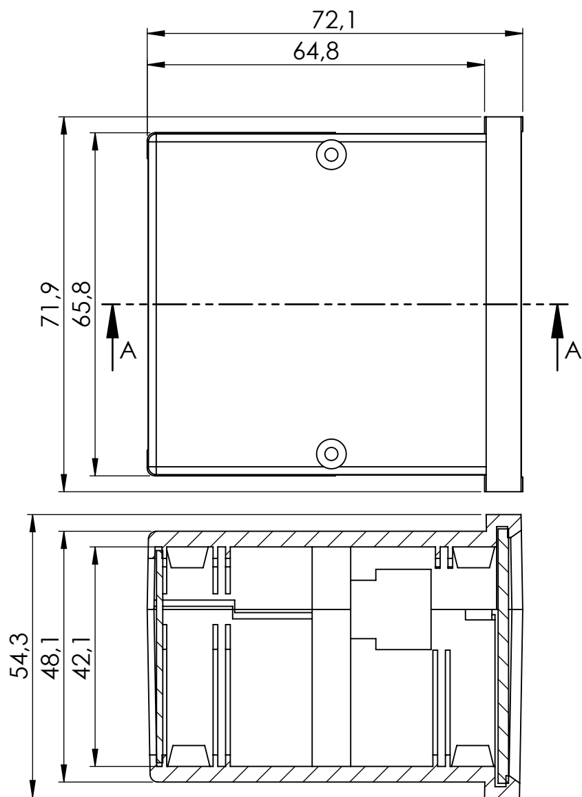
SECTION A-A
