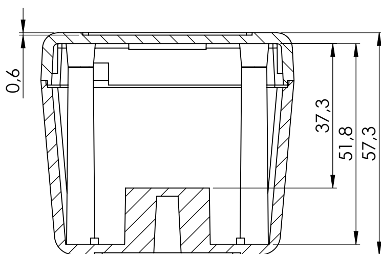
SECTION A-A
