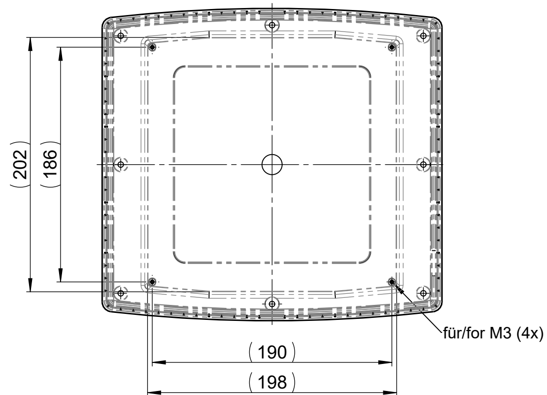
Oberschale (Außenansicht) Top shell (external view)
