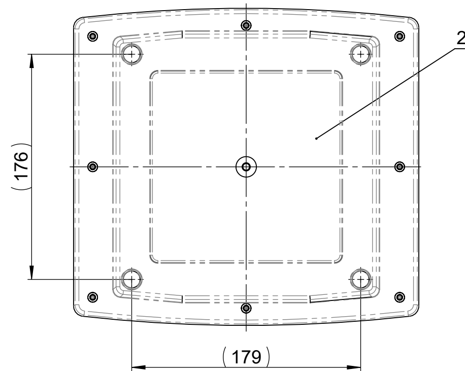
Unterschale (Außenansicht) Bottom shell (external view)
