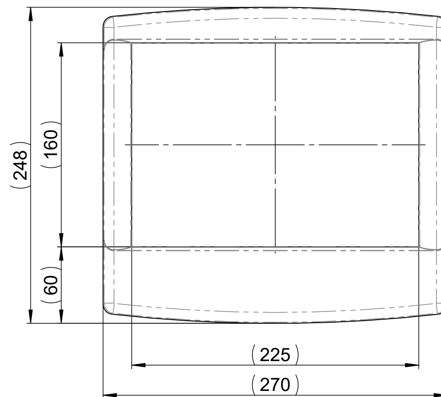
Oberschale (Außenansicht) Top shell (external view)
