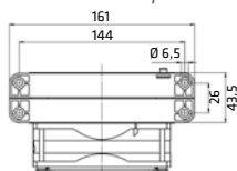
Montaż śrubowy
