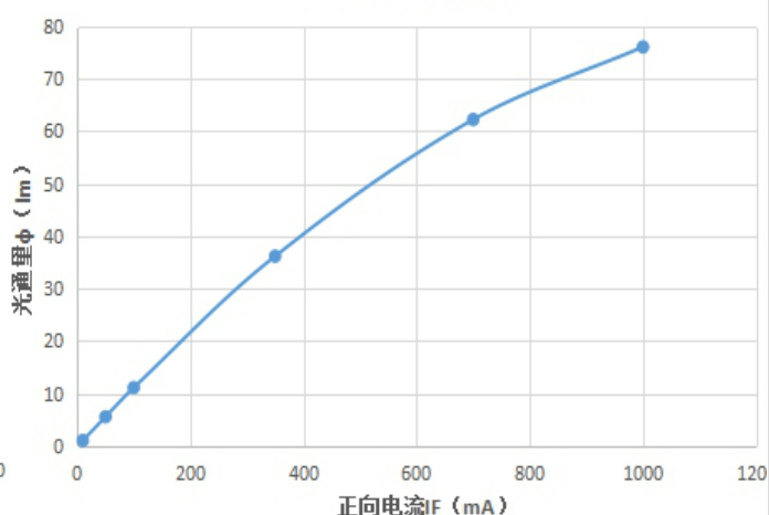
IF- \phi 特性曲线图
