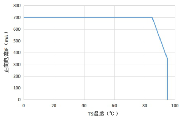
TS-IF特性曲线
