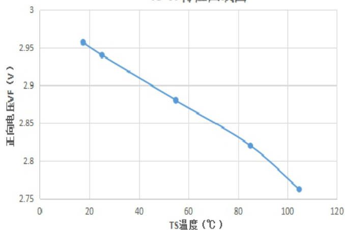
TS-VF特性曲线图
