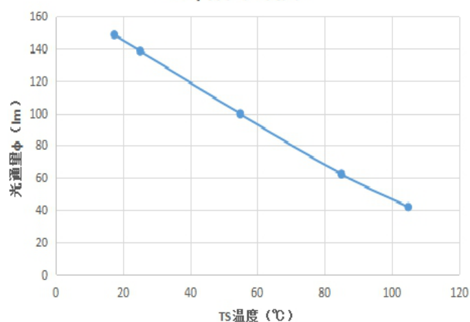
TS- \phi 特性曲线图
