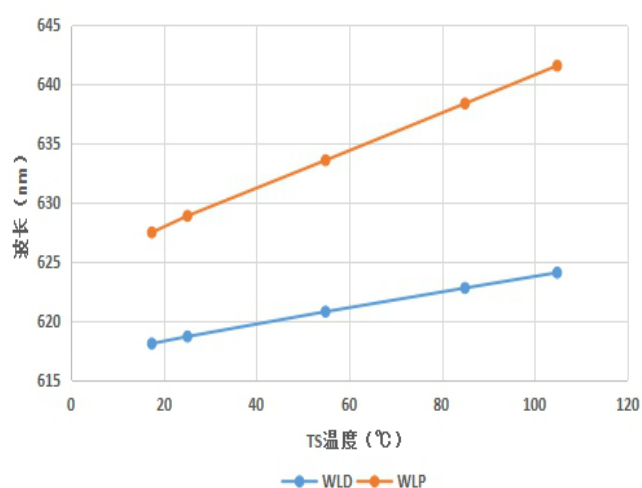
TS-WLD/WLP特性曲线
