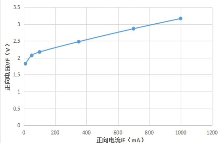
IF-VF特性曲线图
