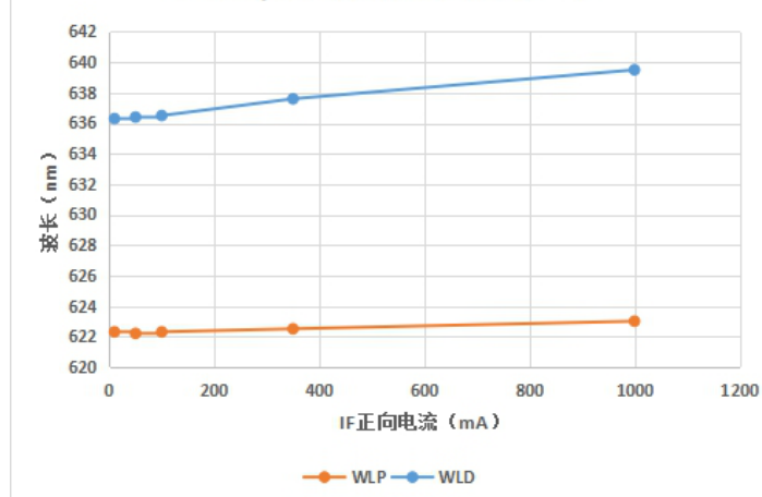
IF-WLD/WLP特性曲线 ( T_s=85^{\circ}\text{C} )
