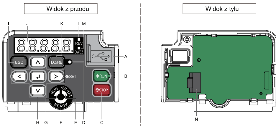
Rysunek 7.1 Klawiatura
