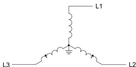
Abbildung 2.7 Symmetrische Erdung
