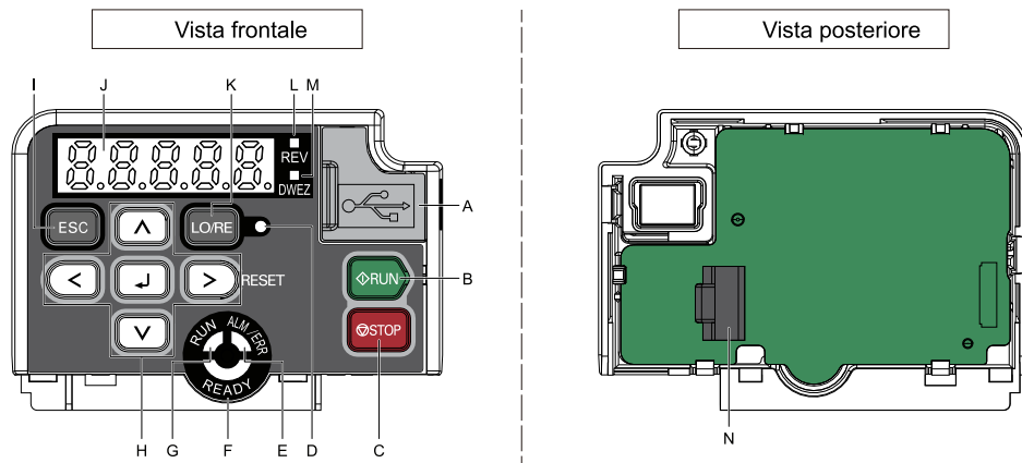
Figura 4.1 Tastiera
