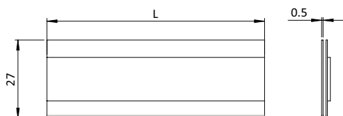
Magnetic Label Holder 27 - 1.06" Magnetischer Einsteckträger 27
