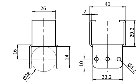
Mounting Bracket ST D28 Montagehalter ST D28
