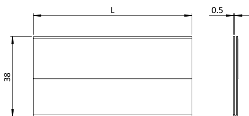
Self-adhesive Label Holder 38 - 1.5" Selbstklebender Einsteckträger 38
