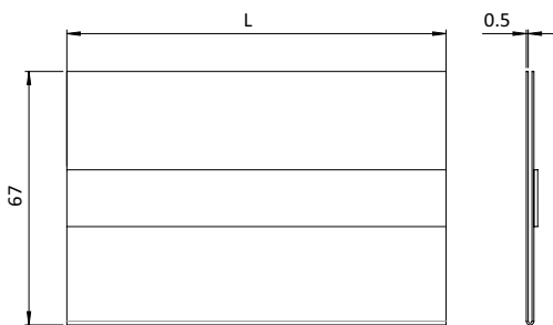
Magnetic Label Holder 67 - 2.64" Magnetischer Einsteckträger 67
