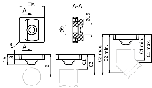
Adapter Plate D28 Adapterplatte D28
