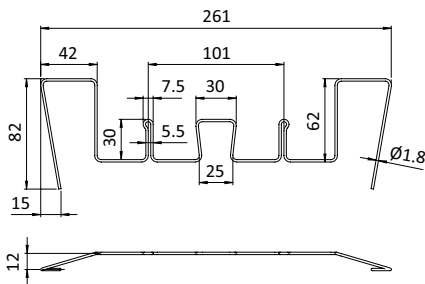
SLC Wire Steel Clamp for Visual Pocket KLT-Drahtbügel für Sichttasche
