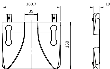
Infeed Cap for Guiding Rail FIFO (Set) Einführungskappe für Führungsschiene FIFO (Set)
