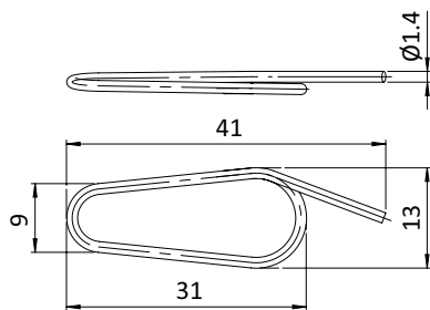
U-loop Steel Clamp for Visual Pocket Bügelklemme für Sichttasche
