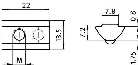
Roll-in T-slot Nut 13.5 x 7.2 mm with Spring Loaded Ball Nutenstein 13,5 x 7,2 mm, einschwenkbar mit Federkugel
