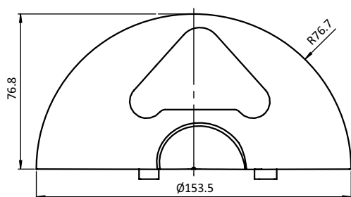
End Cap for Parking Rail Low / High (Set) Endkappe für Parkschiene flach / hoch (Set)
