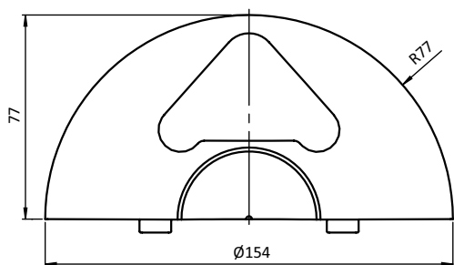
End Cap for Parking Rail High / High (Set) Endkappe für Parkschiene hoch / hoch (Set)
