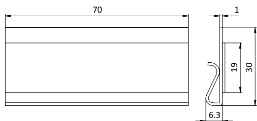
KANBAN Clip Document Holder 70 x 30 - 2.8" x 1.2" KANBAN-Clip Dokumentenhalter 70 x 30
