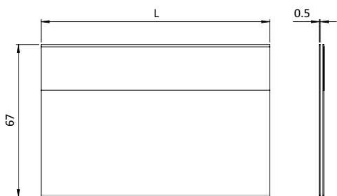
Self-adhesive Label Holder 67 - 2.64" Selbstklebender Einsteckträger 67
