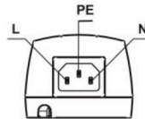
Rys. 2 Układ wyprowadzeń gniazda wejściowego IEC320
