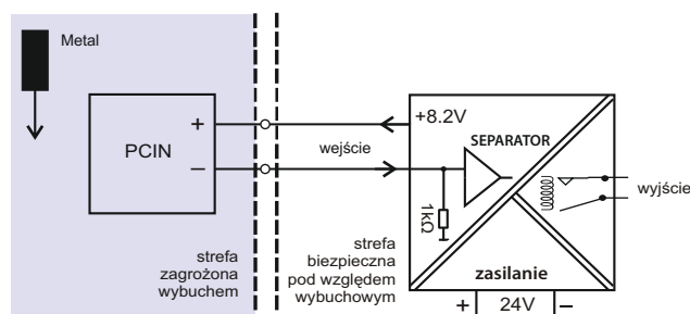
Współpata czujnika PCIN z separatorem
