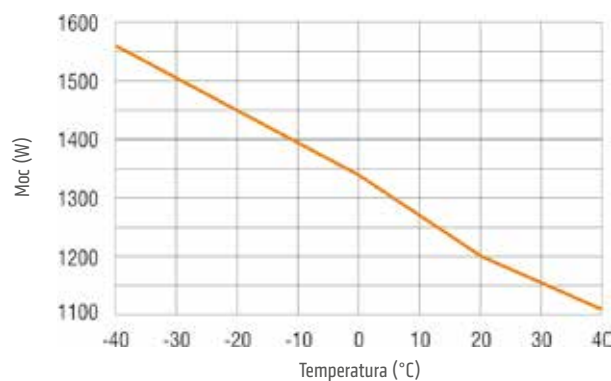
Moc grzewcza / Temperatura otoczenia CS 130
