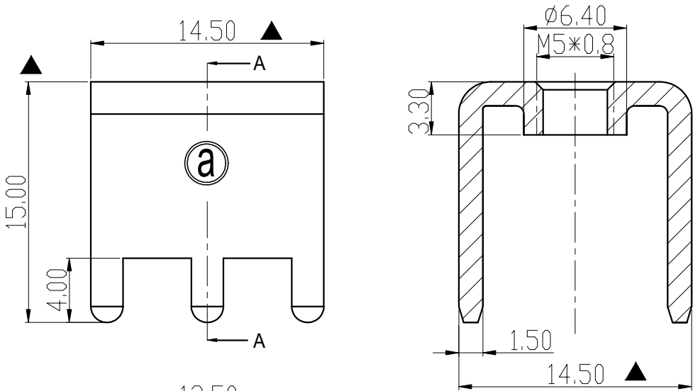
SECTION A-A
