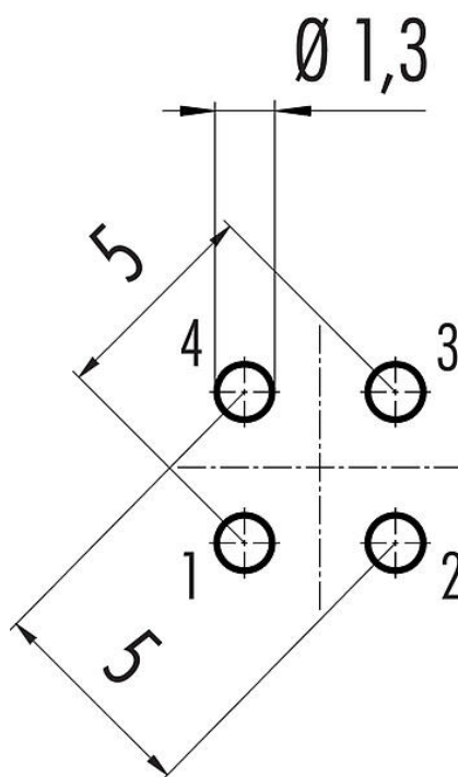
Układ przewodów
