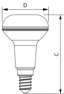
R50 3-25W 105lm 36D 2700K E14 No
