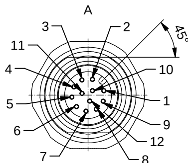
PIN layout PCB/ Lochbild Leiterplatte
