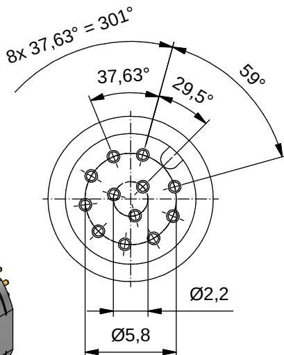
PIN layout PCB/ Lochbild Leiterplatte
