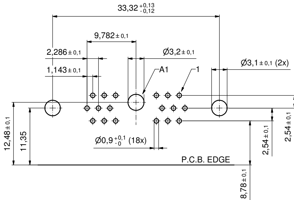
P.C.B. HOLE DRILLINGS ( P.C.B. TOP SIDE )
