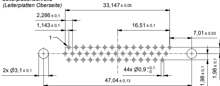
PCB hole drillings (PCB top side)/ Leiterplattenbohrbild (Leiterplatten Oberseite)
