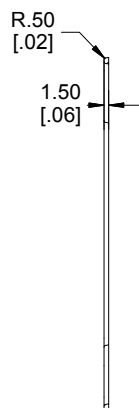
SECTION A-A
