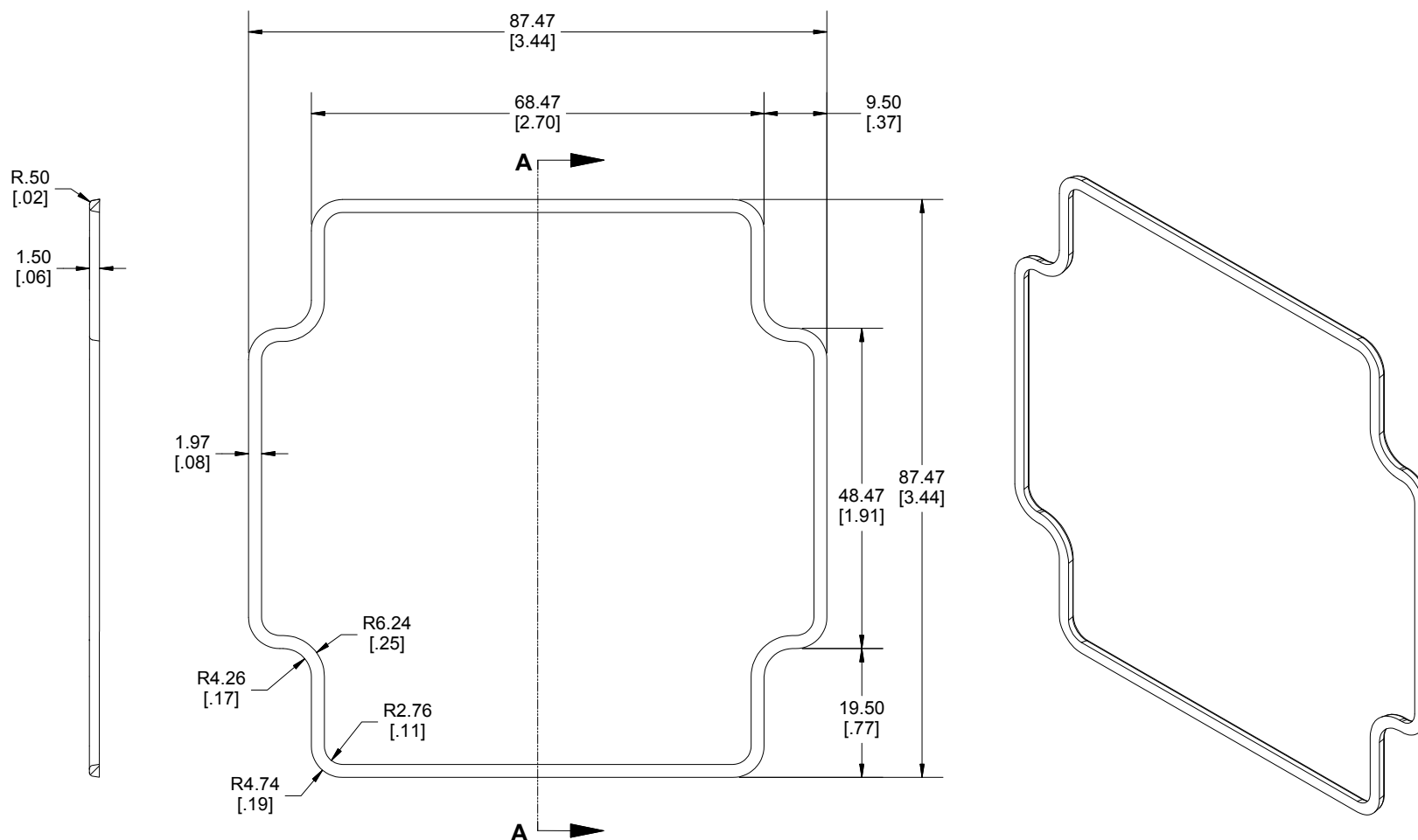
SECTION A-A
