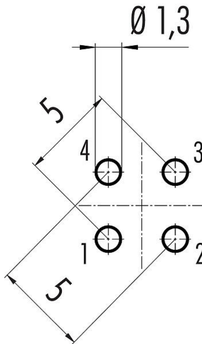
Układ przewodów
